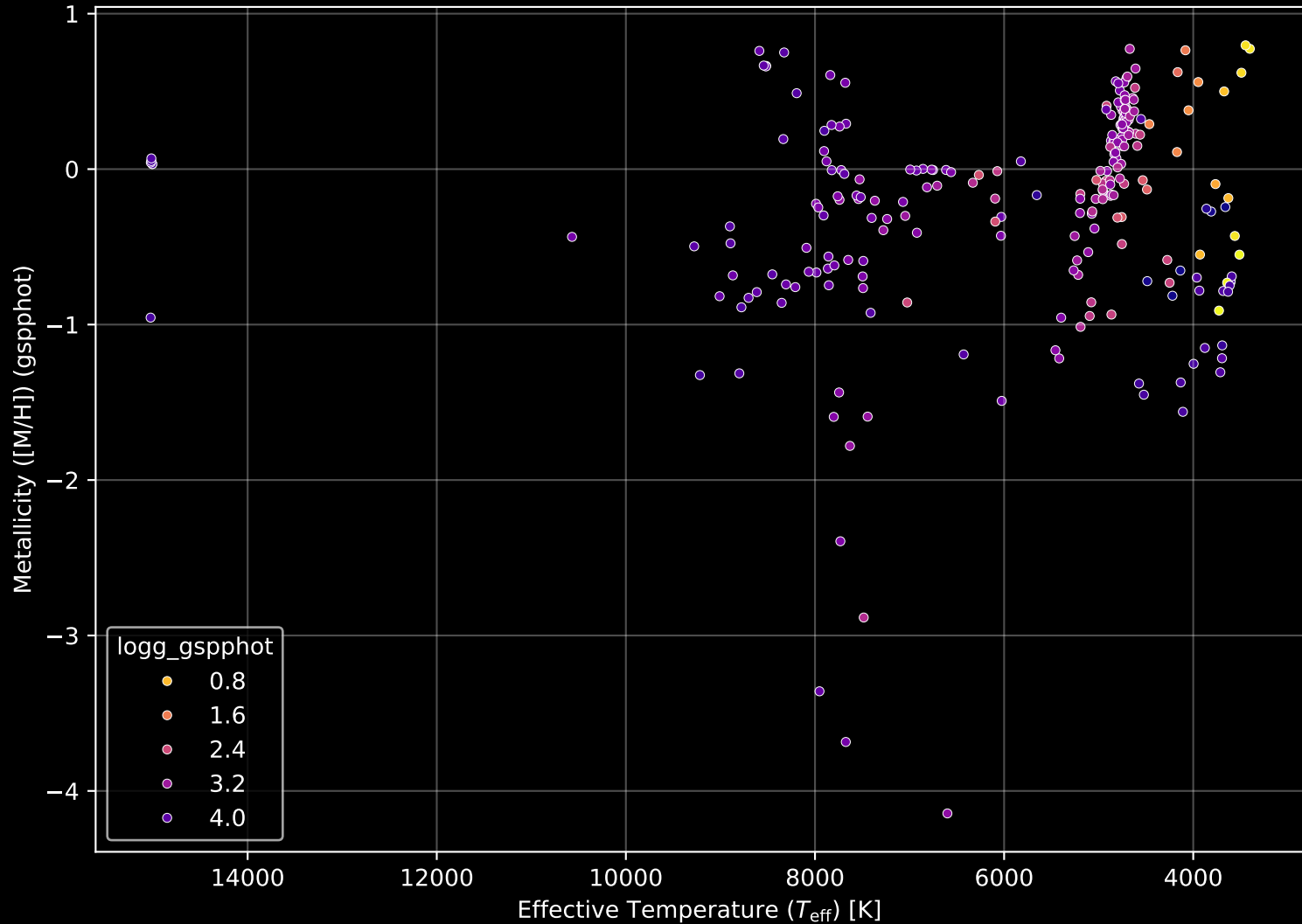
APOGEE DR17 Field: [000+04-O] Stellar Population Parameters (n= 246)
